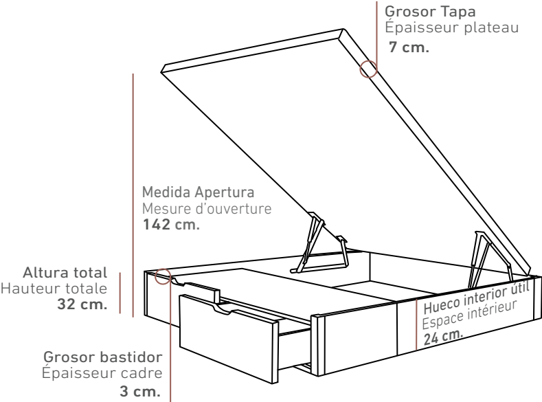
Vista lateral (Las medidas pueden variar ±1cm.) Las medidas de 90 y 105 cm. de ancho se fabrican con 1 cajón. Vue latérale (Les mesures peuvent varier de ±1 cm.) Les mesures en 90 et 105 cm. de large seront fabriqués avec 1 tiroir.
