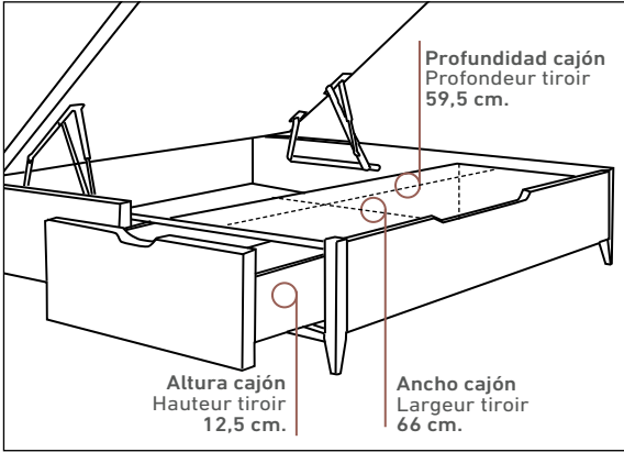
Medida cajones para canapé de 150 cm. Mesure tiroirs pour lit coffre de 150 cm.
