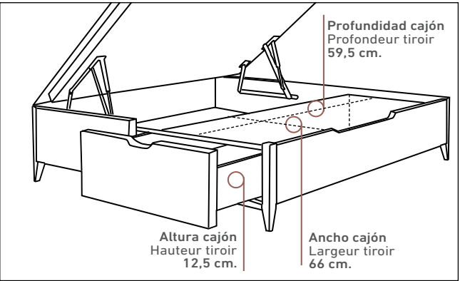
Medida cajones para canapé de 150 cm. Mesure tiroirs pour lit coffre de 150 cm.
