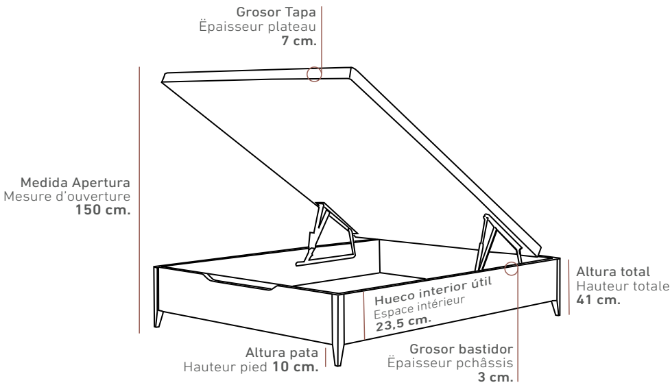
Vista lateral (Las medidas pueden variar \pm 1 cm.) Vue latérale (Les mesures peuvent varier de \pm 1 cm.) 6 patas de refuerzo en el fondo del canapé 6 pieds de renfort au bas du lit coffre
