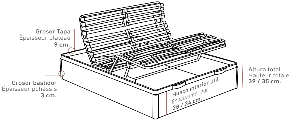
Vista lateral (Las medidas pueden variar ±1 cm.) Vue latérale (Les mesures peuvent varier de ±1 cm.)
