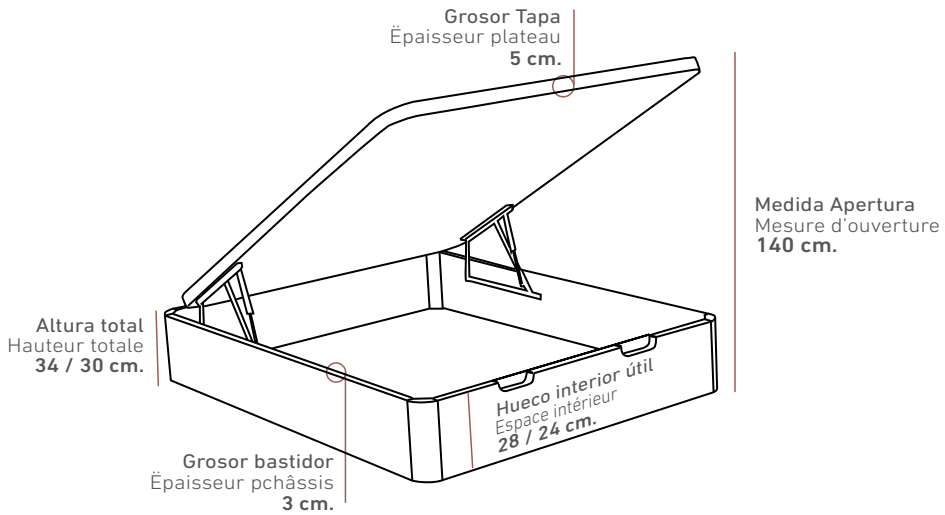
Vista lateral (Las medidas pueden variar \pm 1 cm.) Vue latérale (Les mesures peuvent varier de \pm 1 cm.)
