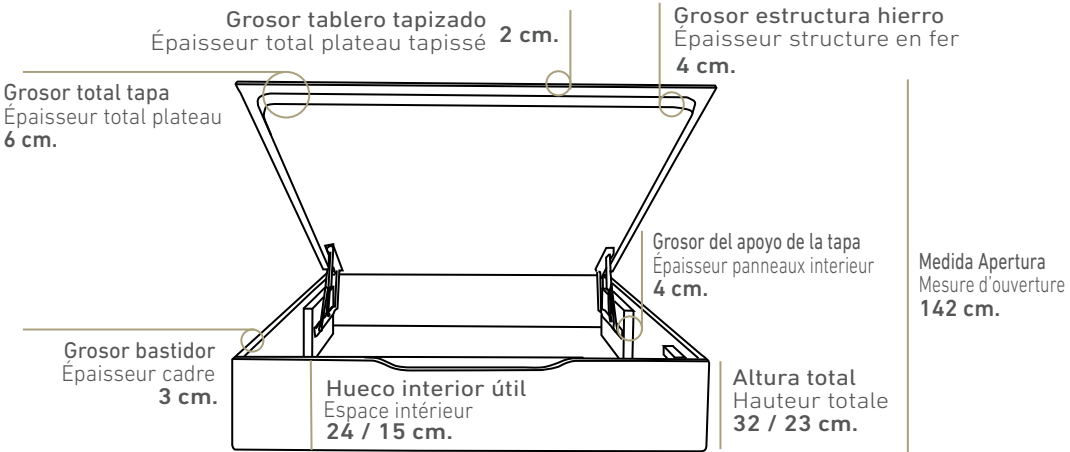
Vista lateral (Las medidas pueden variar ±1cm.) Vue latérale (Les mesures peuvent varier de ±1 cm.)
