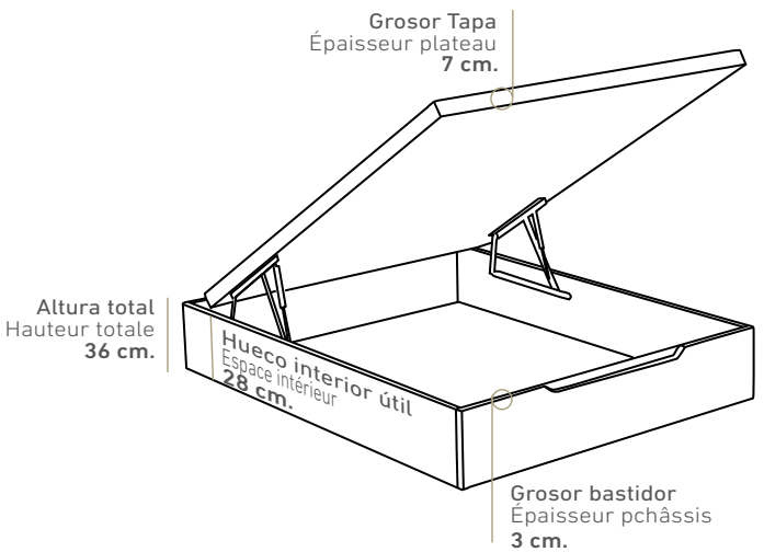
Vista lateral (Las medidas pueden variar ±1cm.) Vue latérale (Les mesures peuvent varier de ±1 cm.)
