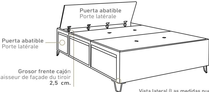
Vista lateral (Las medidas pueden variar ±1cm.) Vue latérale (Les mesures peuvent varier de ±1 cm.)
