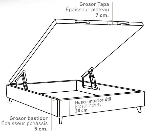
Vista lateral (Las medidas pueden variar ±1cm.) Vue latérale (Les mesures peuvent varier de ±1 cm.)
