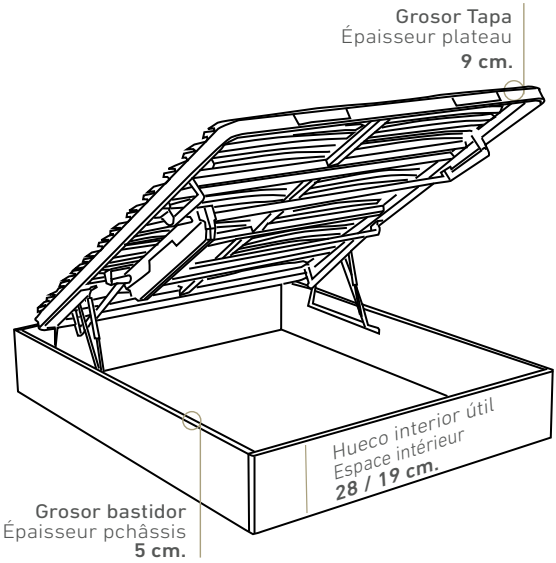
Vista lateral (Las medidas pueden variar ±1cm.) Vue latérale (Les mesures peuvent varier de ±1 cm.)
