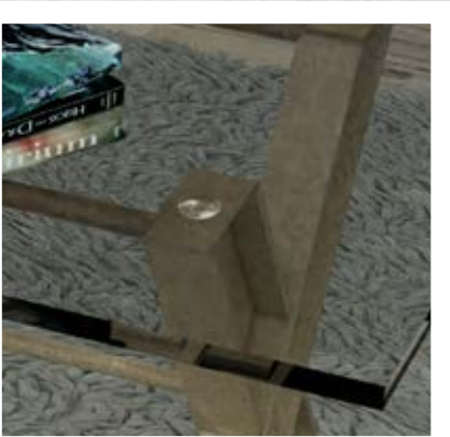
Cogida del cristal al hierro por medio de una ventosa transparente.
