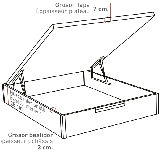
Medida Apertura Mesure d'ouverture 140 cm.
