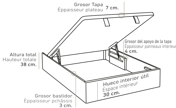
Vista lateral (Las medidas pueden variar ±1cm.) Vue latérale (Les mesures peuvent varier de ±1 cm.)
